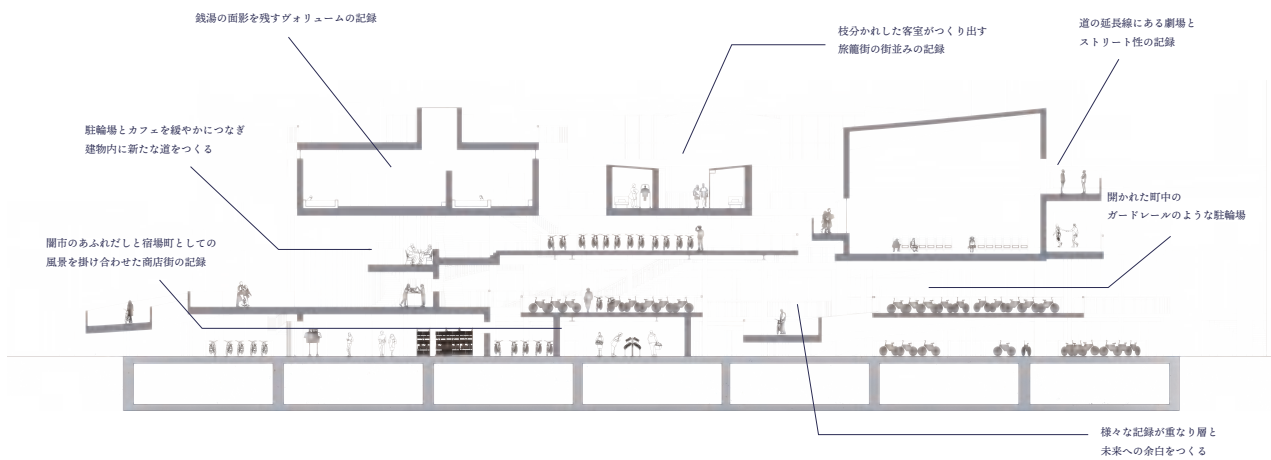
断面図 S-U/500
